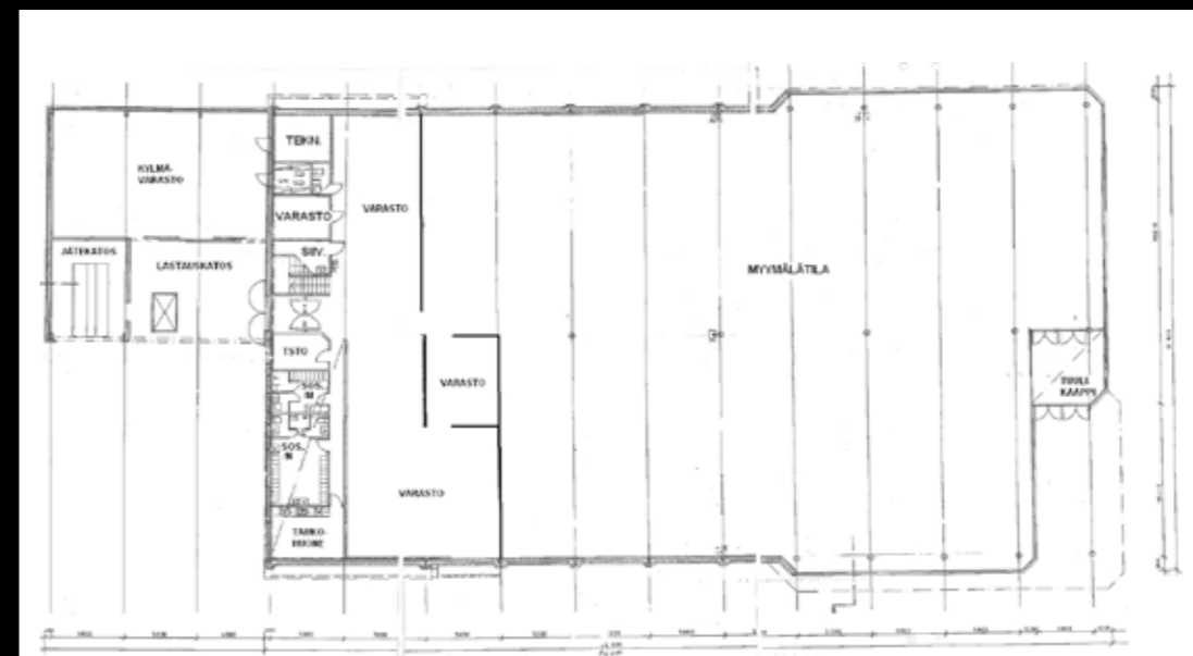
Pohjapiirros
